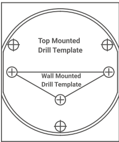
Boorsjabloon (×1)
